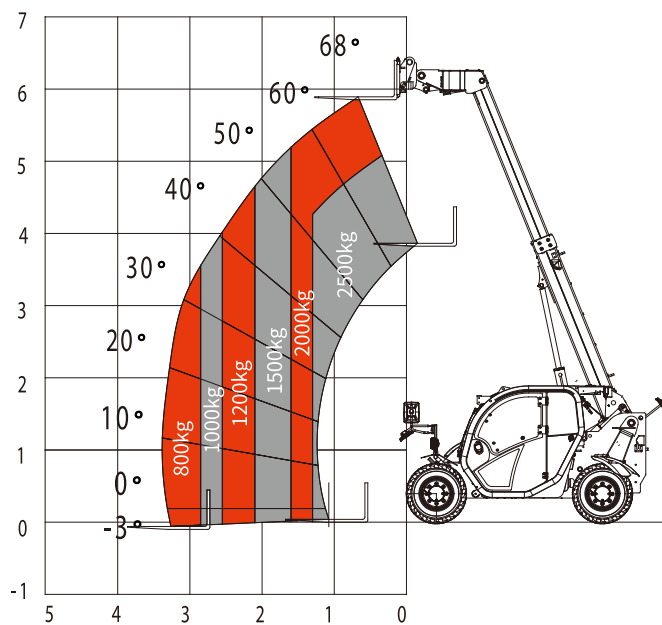
25THCJ06-KU Lifting diagram
